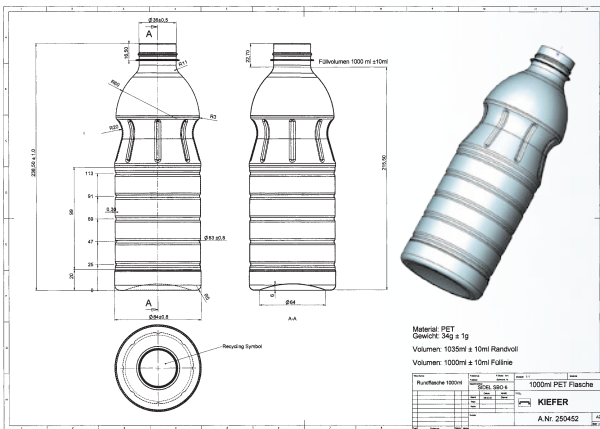
Einfach-Blasform, Rundläufer
